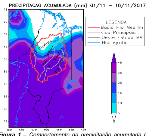
Figura 1 – Comportamento da precipitação acumulada (mm) na extensão da bacia do rio Mearim. Fonte de dados: CPC/NCEP/ANA; Elaboração: TED SUDAM/UFPA/2017.
