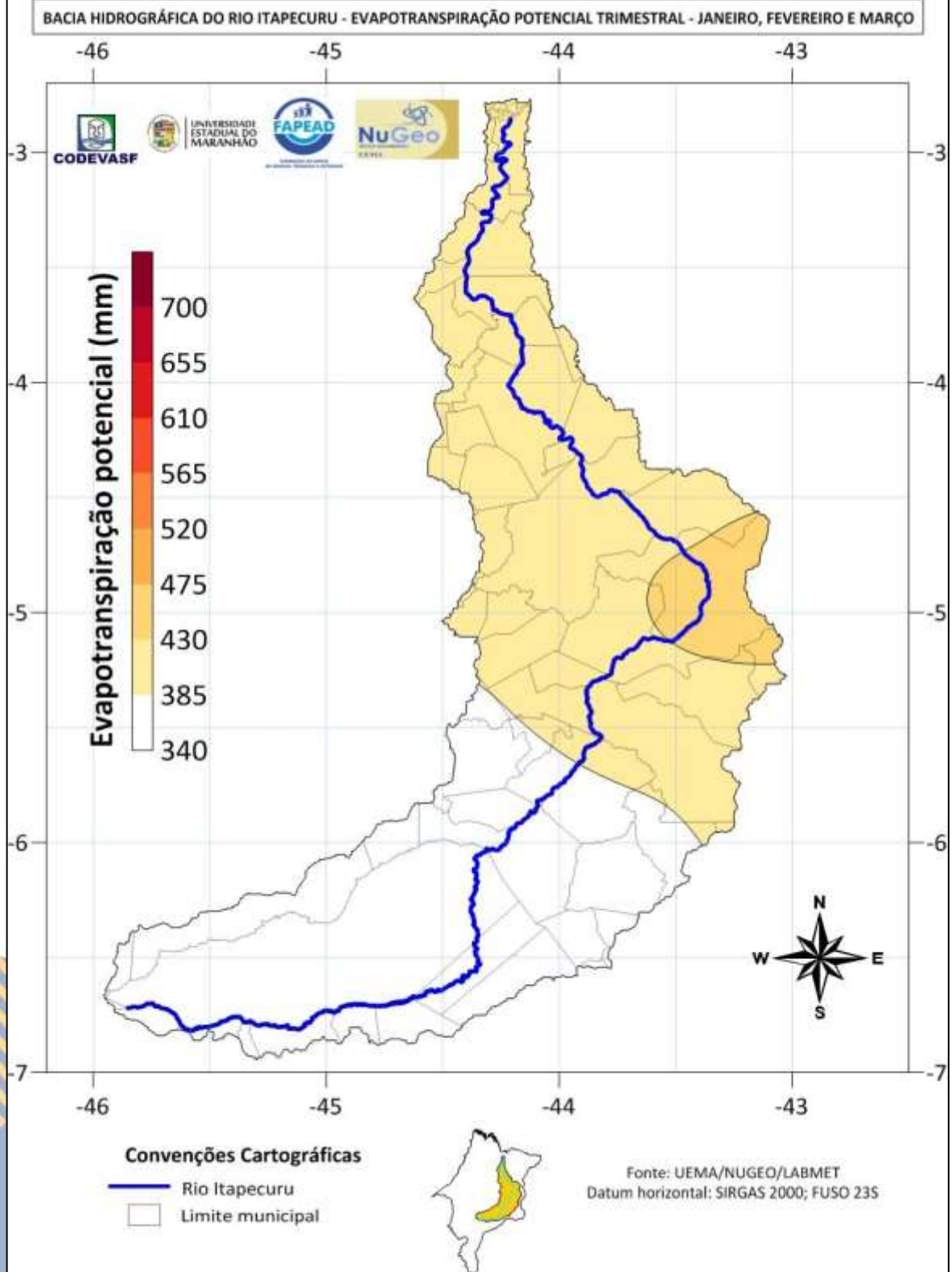
Figura 95 – Evapotranspiração Potencial no trimestre janeiro-fevereiro-março na Bacia do Rio Itapecuru.
