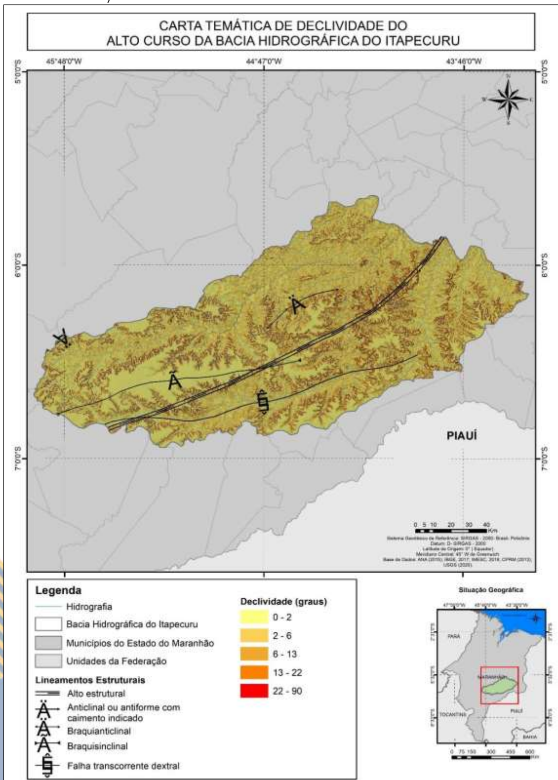
Figura 35 – Cartografia temática de Declividade da Bacia do Alto Curso do Rio Itapecuru (Maranhão, Nordeste do Brasil).
