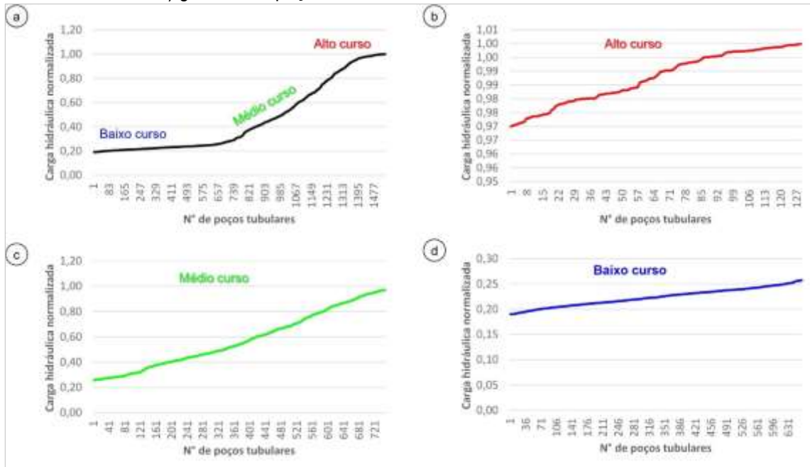
Figura 61 – Avaliação da carga hidráulica ( h ) dos 1.540 poços tubulares no Estado do Maranhão: a) gráfico de h normalizado de todos os poços tubulares, com destaque para os trechos alto, médio e baixo curso; b) gráfico dos poços com 349 \text{ m} < h \leq 580 \text{ m} normalizados; c) gráfico dos poços com 28 \text{ m} < h \leq 349 \text{ m} normalizados; d) gráfico dos poços com h \leq 28 \text{ m} normalizados.
