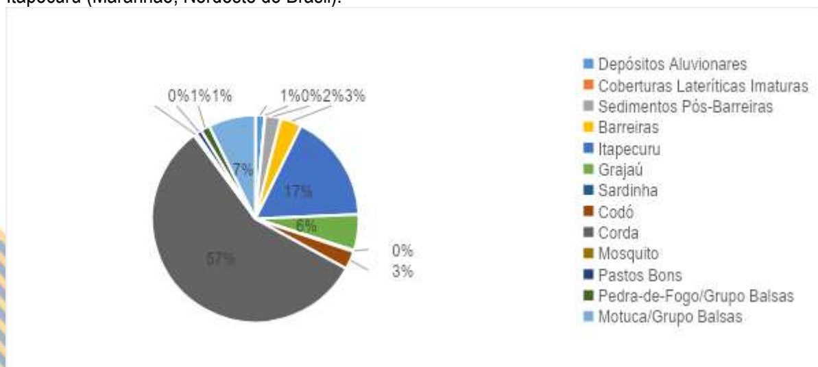
Figura 29 – Gráfico de distribuição areal (km 2 ) das fácies sedimentares na Bacia do Médio Curso do Rio Itapecuru (Maranhão, Nordeste do Brasil).
