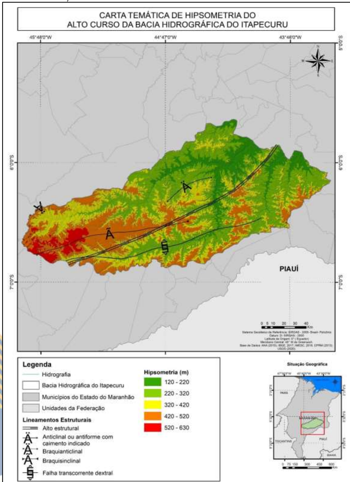
Figura 34 – Cartografia temática de Hipsometria da Bacia do Alto Curso do Rio Itapecuru (Maranhão, Nordeste do Brasil).
