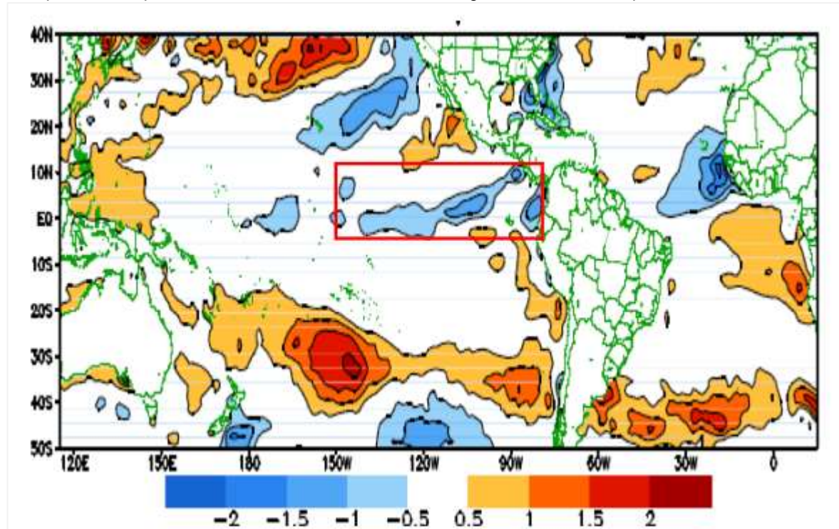
Figura 113 – Anomalias de Temperatura da Superfície do Mar (TSM) para o trimestre fevereiro-março-abril de 2009. A intensidade das anomalias de TSM é em °C. As cores laranja-vermelho indicam águas mais quentes do que o normal e cores em azul indicam águas mais frias do que o normal.
