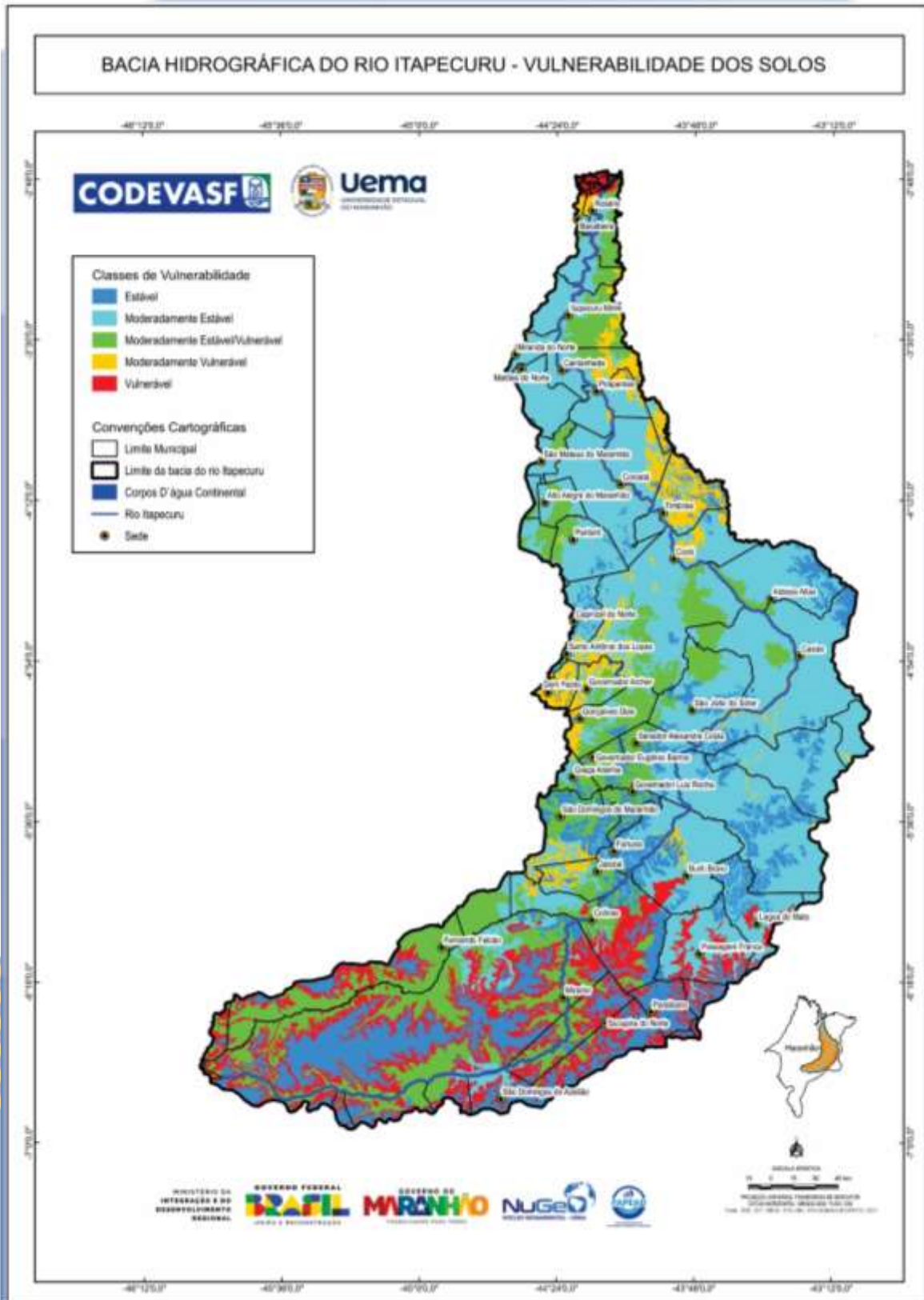
Figura 122 – Mapa de Vulnerabilidade Natural dos solos da bacia hidrográfica do Rio Itapecuru, Estado do Maranhão.
