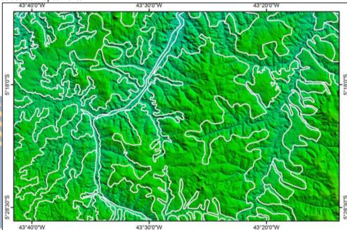
Figura 118 – Imagem de Radar do Projeto TOPODATA com detalhes dos limites das unidades de mapeamento.
