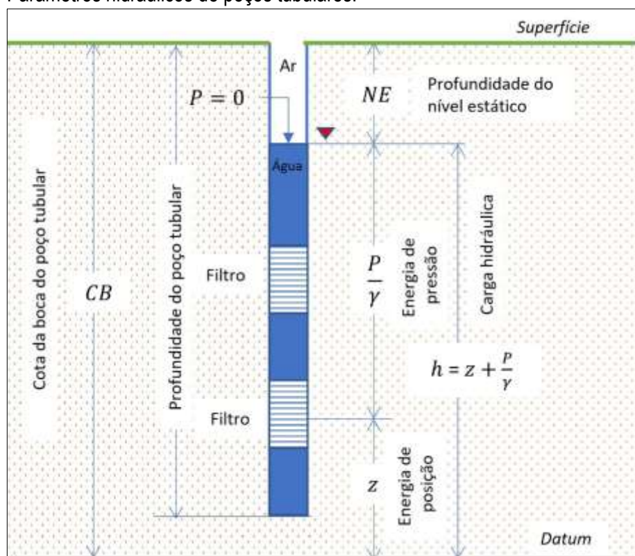
Figura 63 – Parâmetros hidráulicos de poços tubulares.
