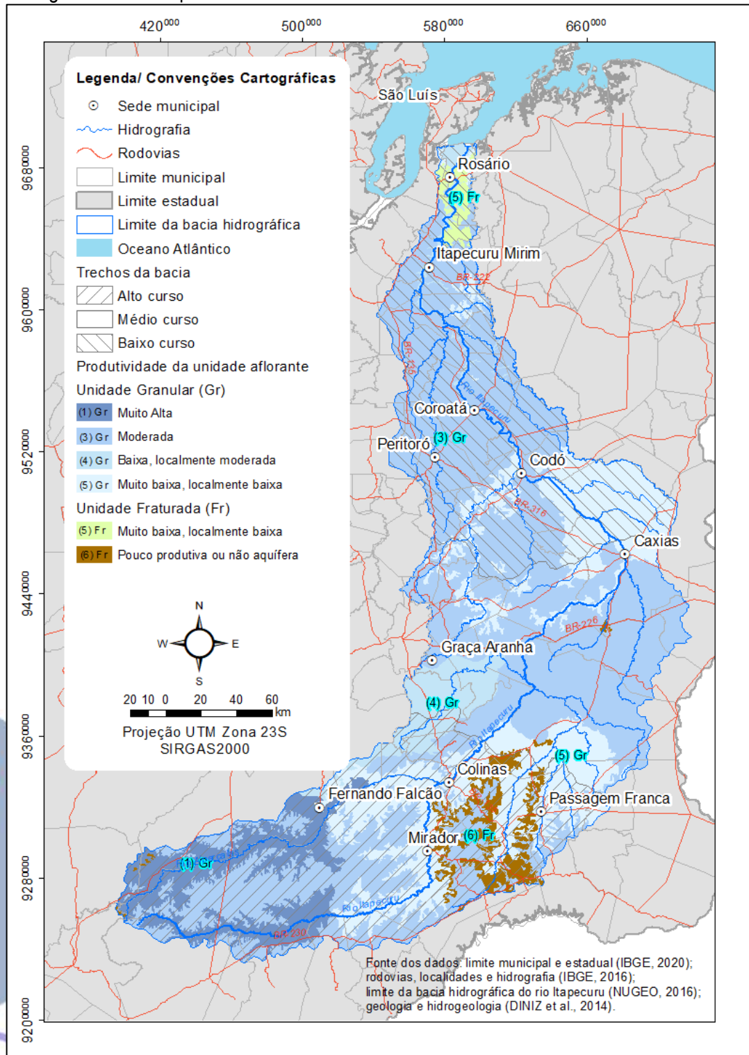
Figura 72 – Mapa temático síntese de produtividade das unidades hidroestratigráficas aflorantes na bacia hidrográfica do rio Itapecuru.
