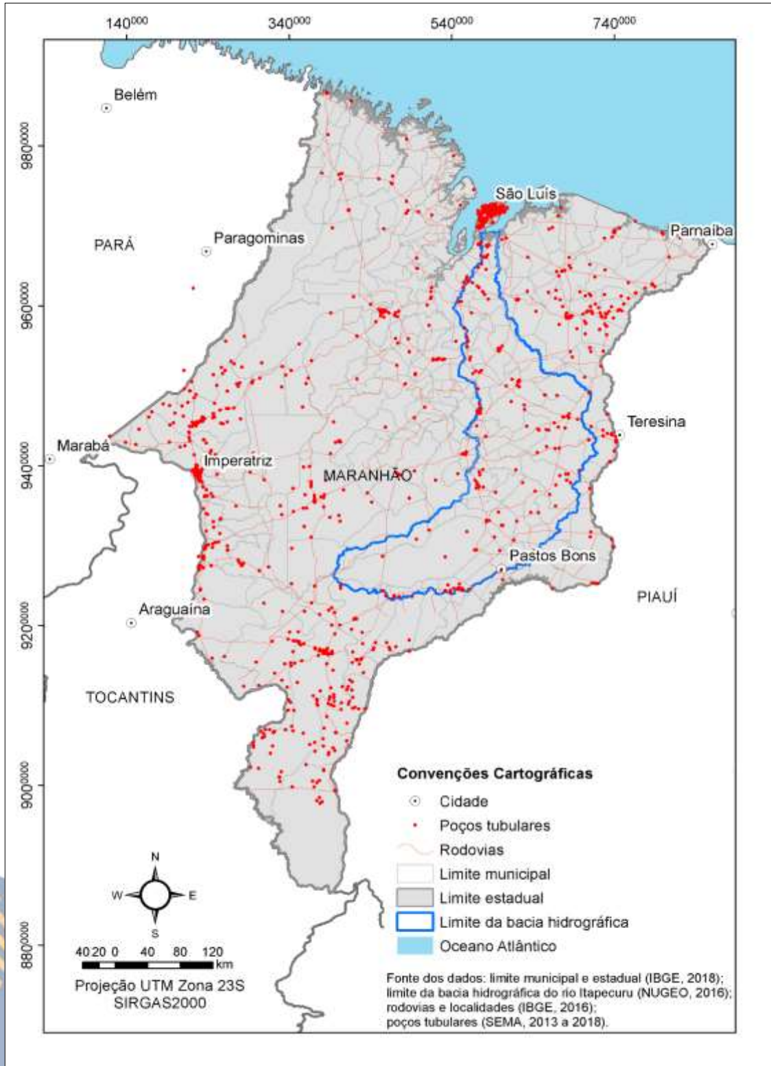
Figura 57 – Mapa temático de distribuição dos 155 poços tubulares segundo o trecho da bacia hidrográfica do rio Itapecuru.
