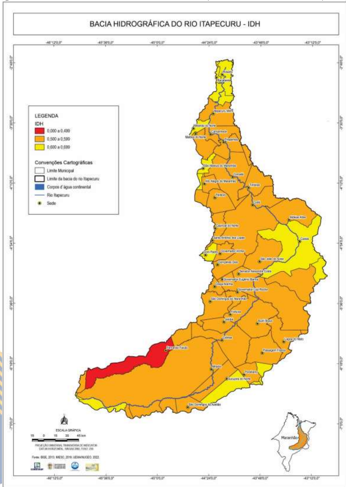
Figura 243 – Índice de Desenvolvimento Humano dos municípios inseridos na Bacia do Rio Itapecuru.
