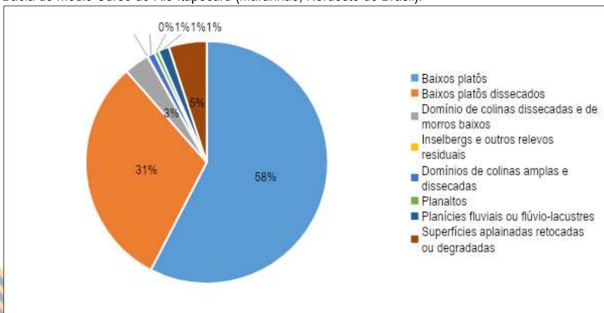
Figura 47 – Gráfico demonstrativo de percentual de área ocupada por unidades geomorfológicas na Bacia do Médio Curso do Rio Itapecuru (Maranhão, Nordeste do Brasil).
