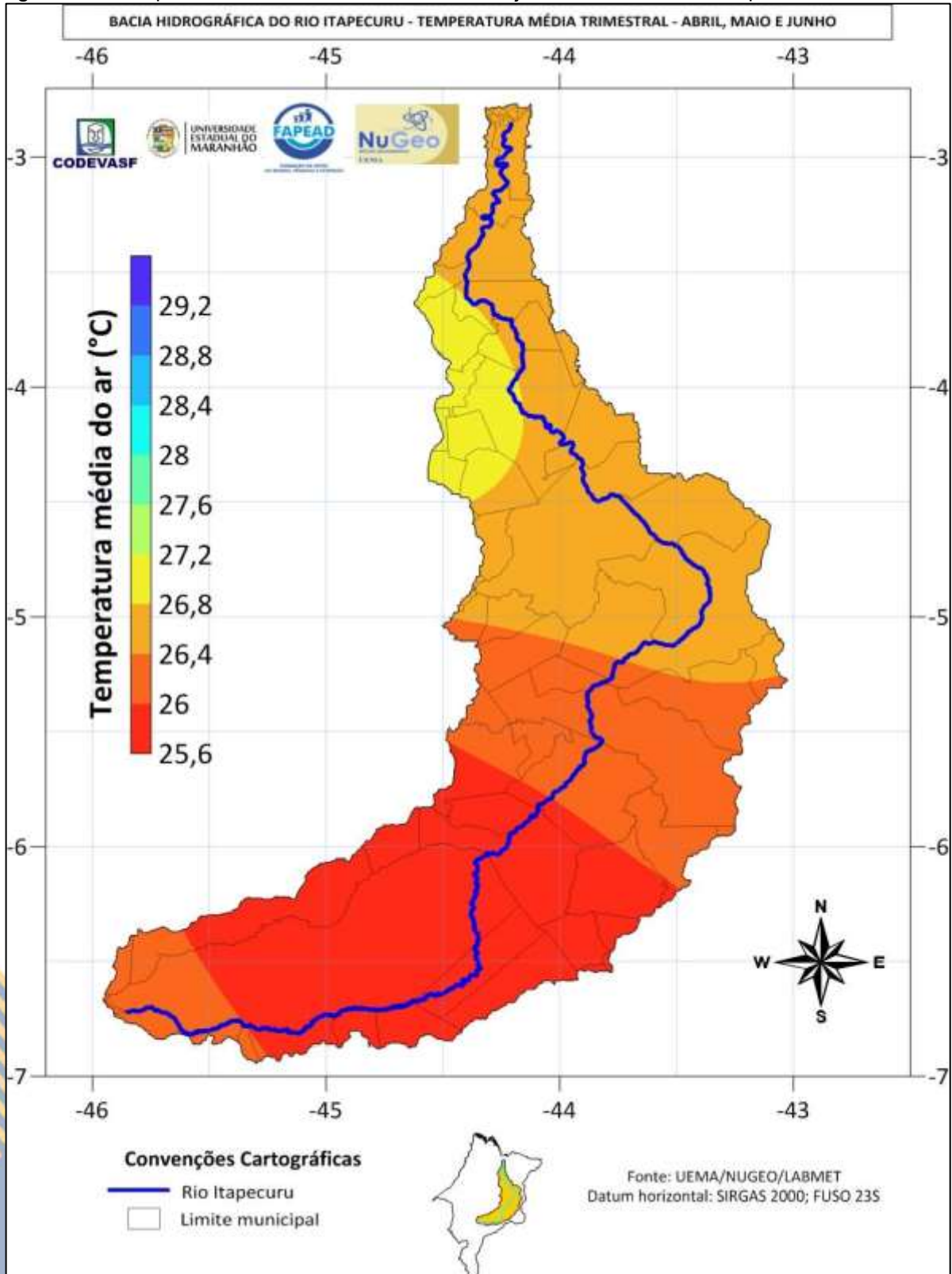
Figura 91 – Temperatura média no trimestre abril-maio-junho na Bacia do Rio Itapecuru.
