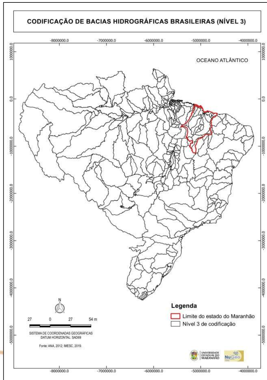
Figura 7: Nível 3 de codificação das bacias hidrográficas brasileiras.
