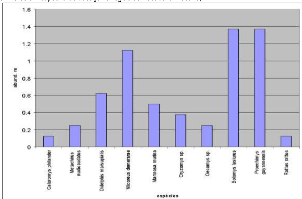
Figura 151 – Abundância relativa (número de indivíduos por 100 armadilhas x noite) de pequenos mamíferos em capoeira de babaçu na região de Bacabeira-Rosário, MA.
